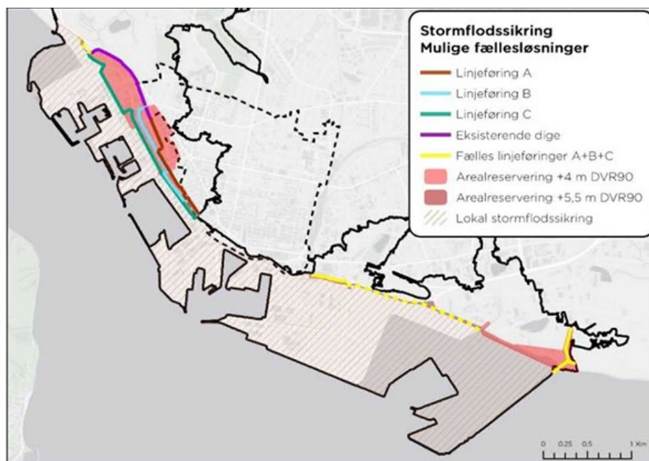
Kort 8.1.2 Muligt løsningsrum – linjeføringer til fælles stormflodssikring af midtbyen. Her ses at dele af lokalplanområdet skal afværges mod oversvømmelse ved terrænregulering til minimumskote, samt at linjeføringen for mulig stormflodssikring skal følge grusvejen mellem Mådevej og kysten i planområdet.
