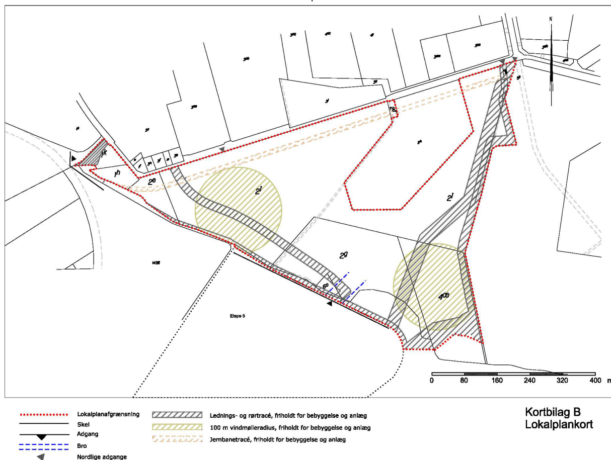
Kort 7.2 Lokalplankort, Lokalplan nr. 11-030-0010 Erhvervsområde syd for Mådevej.
