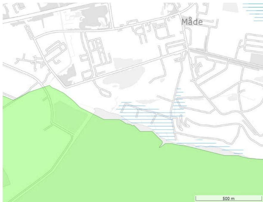
Figur 3.13 - Inden for planområdet er udpeget lavbundsareal (blå skraver) og den sydlige del af planområdet er udpeget med miljømål for kystvand (grøn flade). Nord er op.
